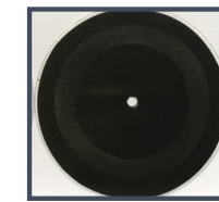
Un coloris plaxé standard noir après 100 cycles d'abrasion : une décoloration apparaît de façon précoce.
