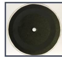
Un coloris plaxé standard noir après 100 cycles d'abrasion : une décoloration clairement visible avec un changement de brillance.
